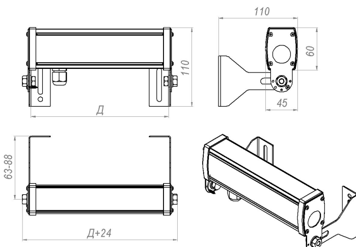
Габаритні розміри.
