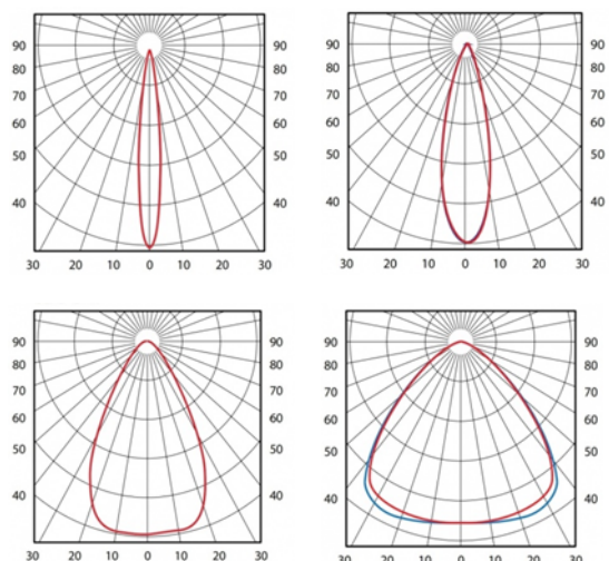
Діаграма КСС.
