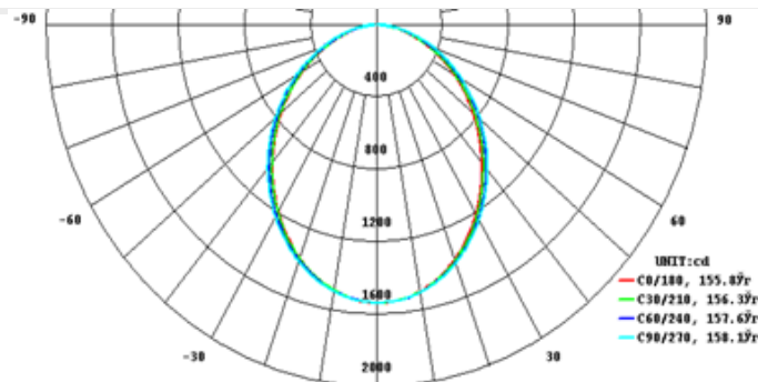
Діаграма КСС.
